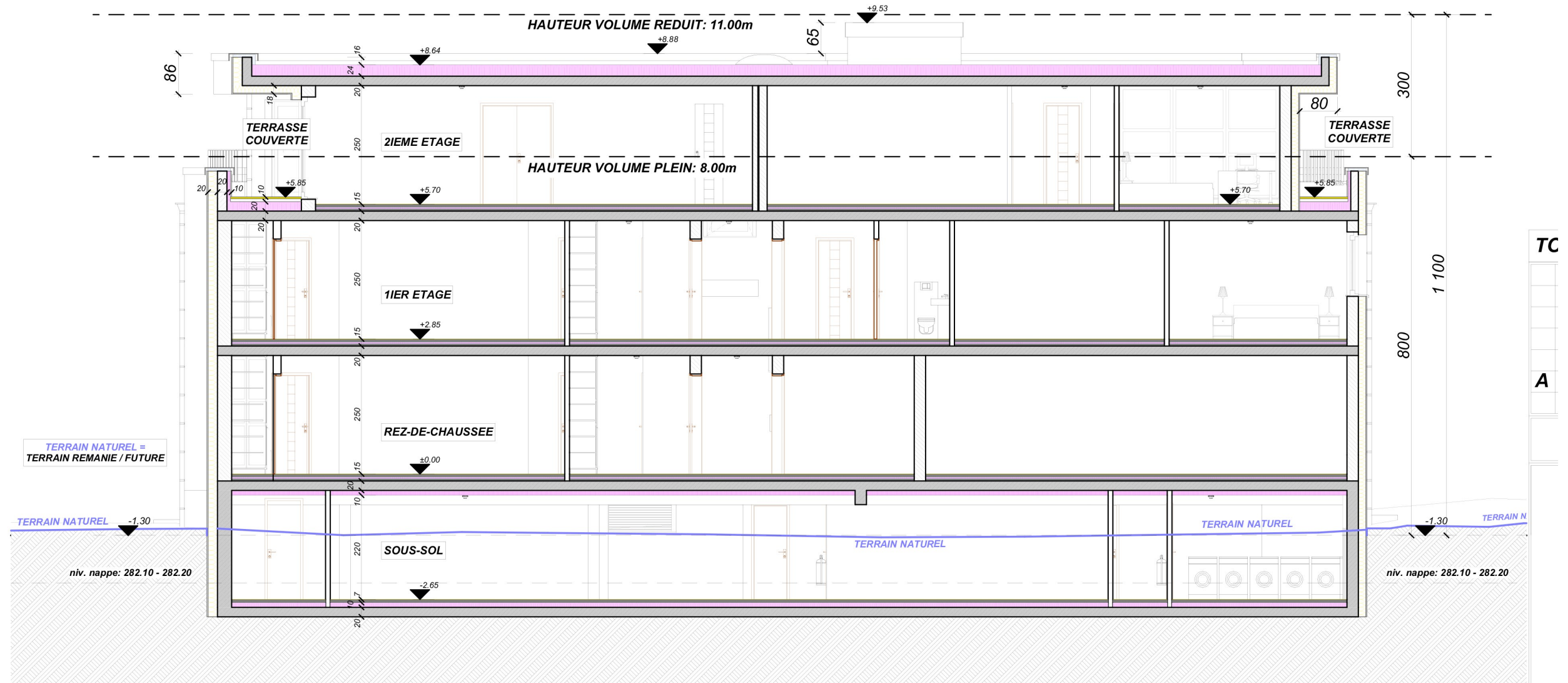
COUPE SCHEMATIQUE (longitudinale)
